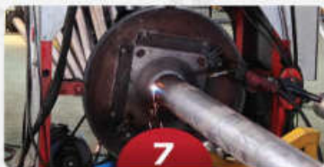
7 Hàn đế trụ đèn Base plate welding process
